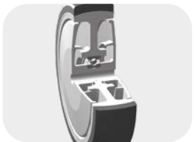
Aufbau Rad: Kugellager abgedichtet
